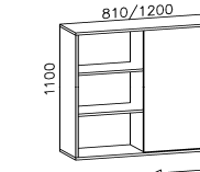
right: sliding door
